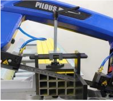
Прижим вертикальный ручной, VP 260
