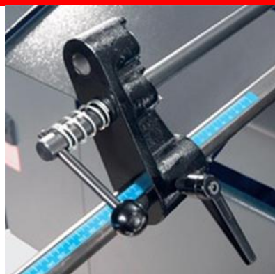
Упор для выставления заготовок со шкалой, длиной 500 мм, DR
