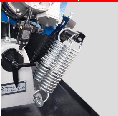
Механическая регулировка угла подъема рамы
